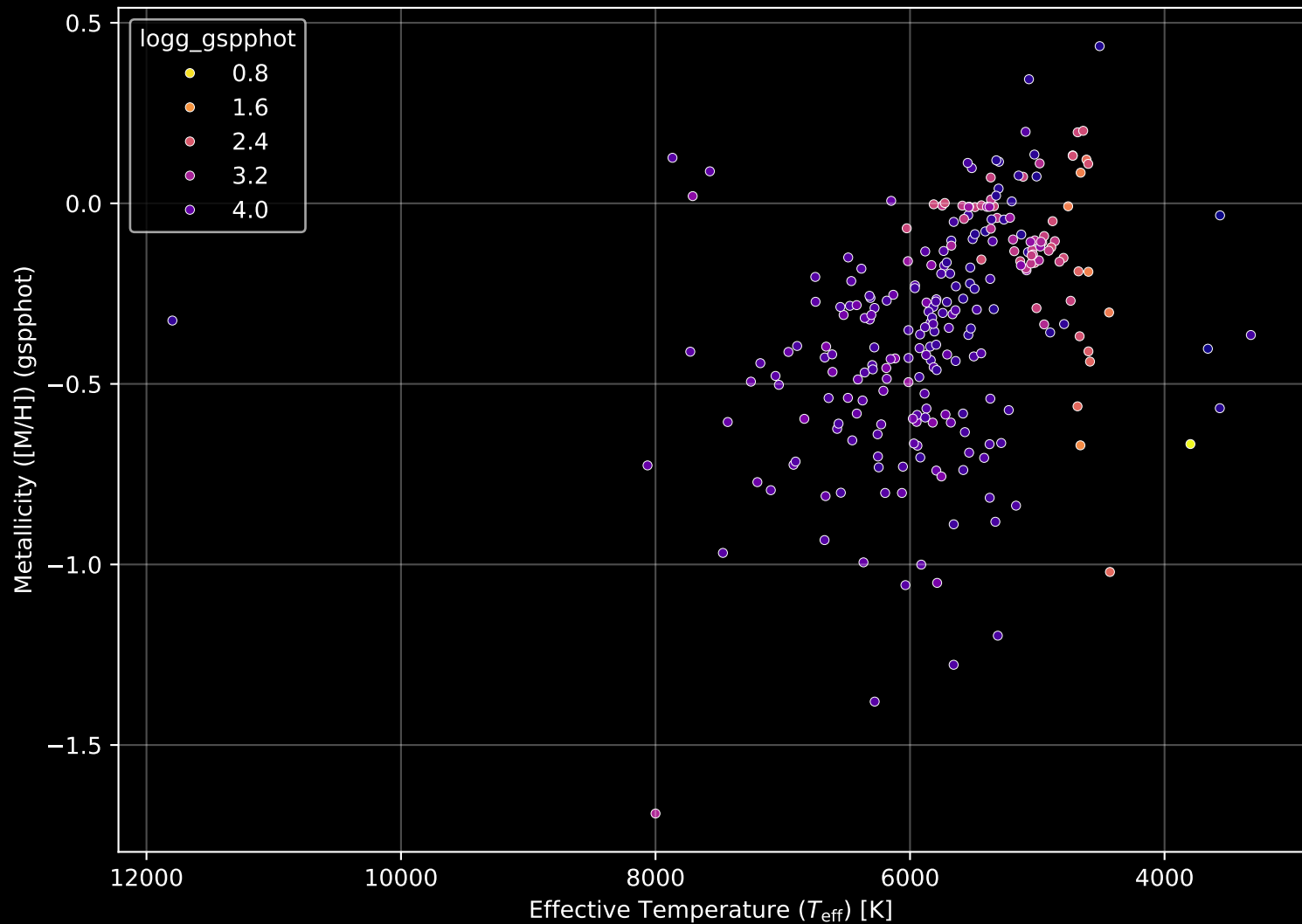
GALAH DR4 Field: [2955] Stellar Population Parameters (n= 251)
