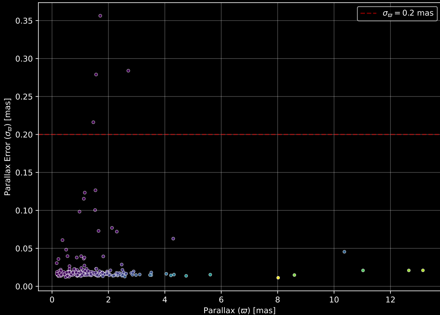
GALAH DR4 Field: [2955] Parallax Quality (n= 251)
