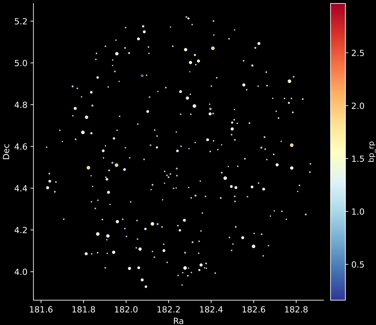
GALAH DR4 Field: [2955] Stars: 251
