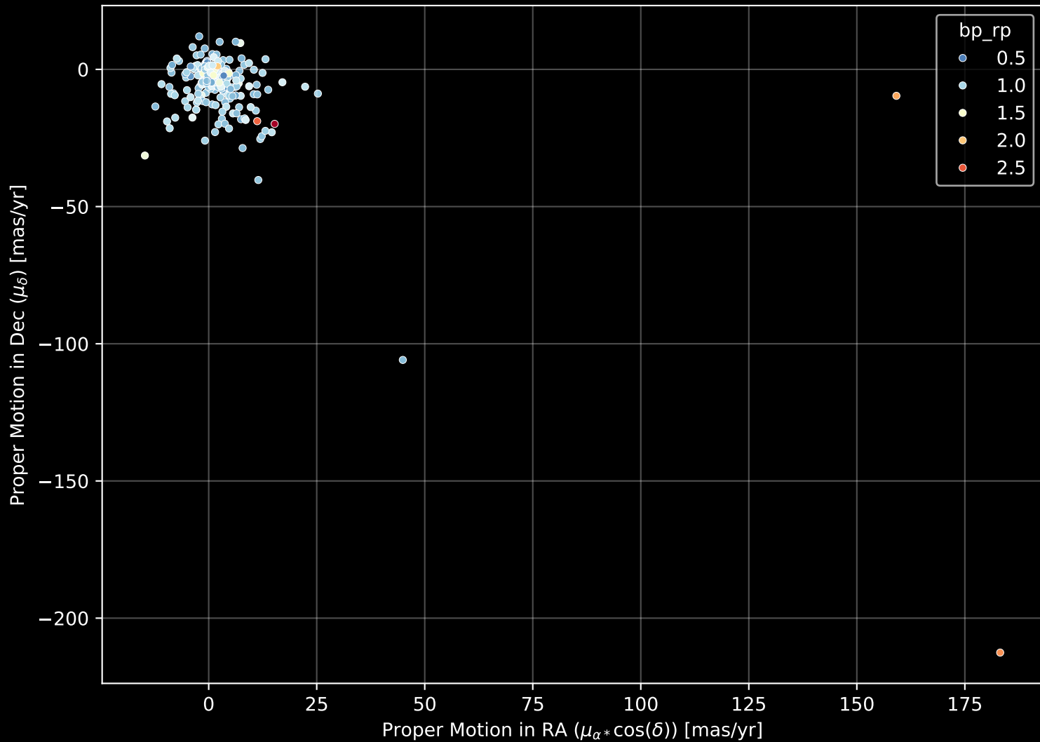
GALAH DR4 Field: [2955] Proper Motion Diagram (n= 251)
