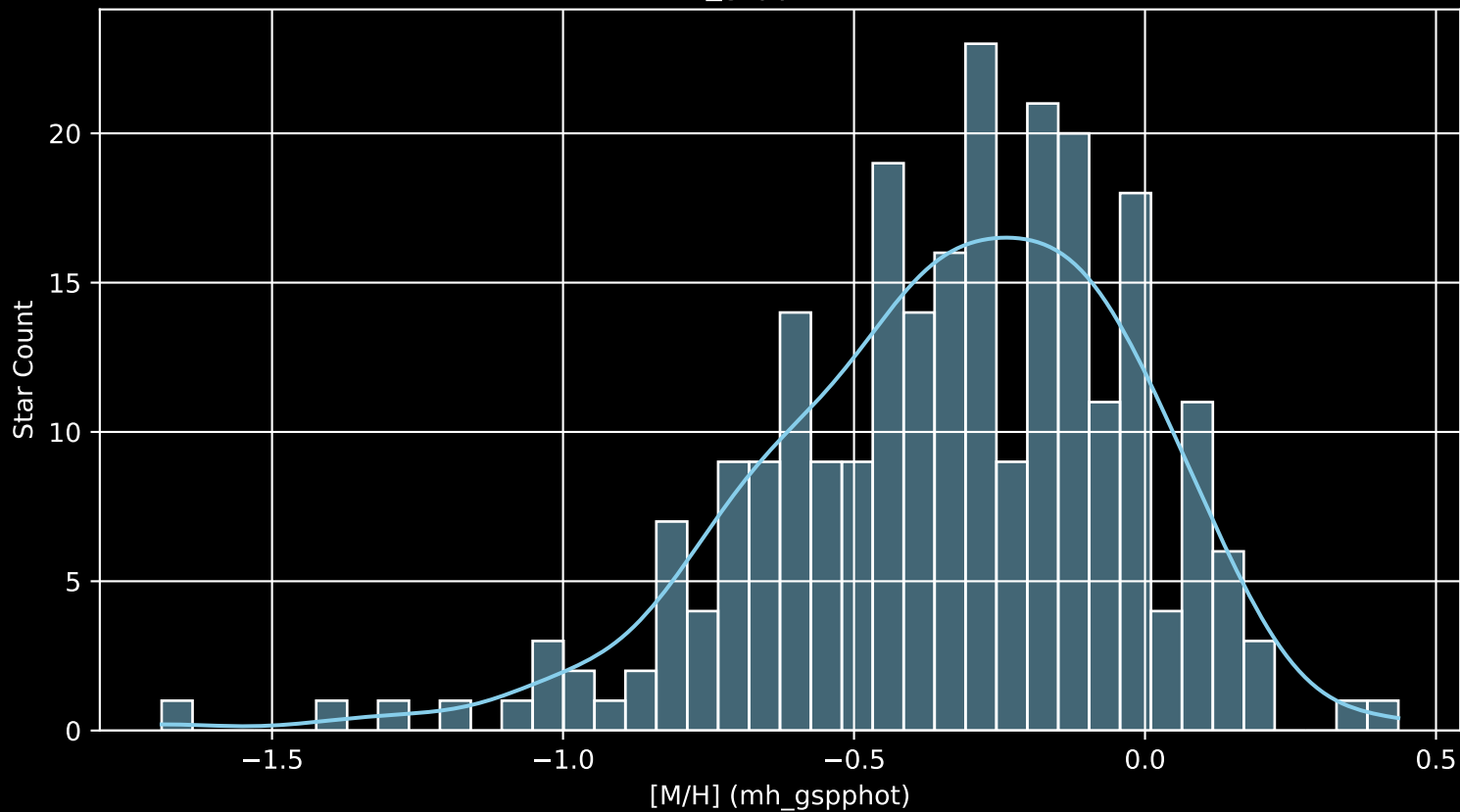
GALAH DR4 Field: [2955] [M/H] (mh_gspphot) (n= 251)
